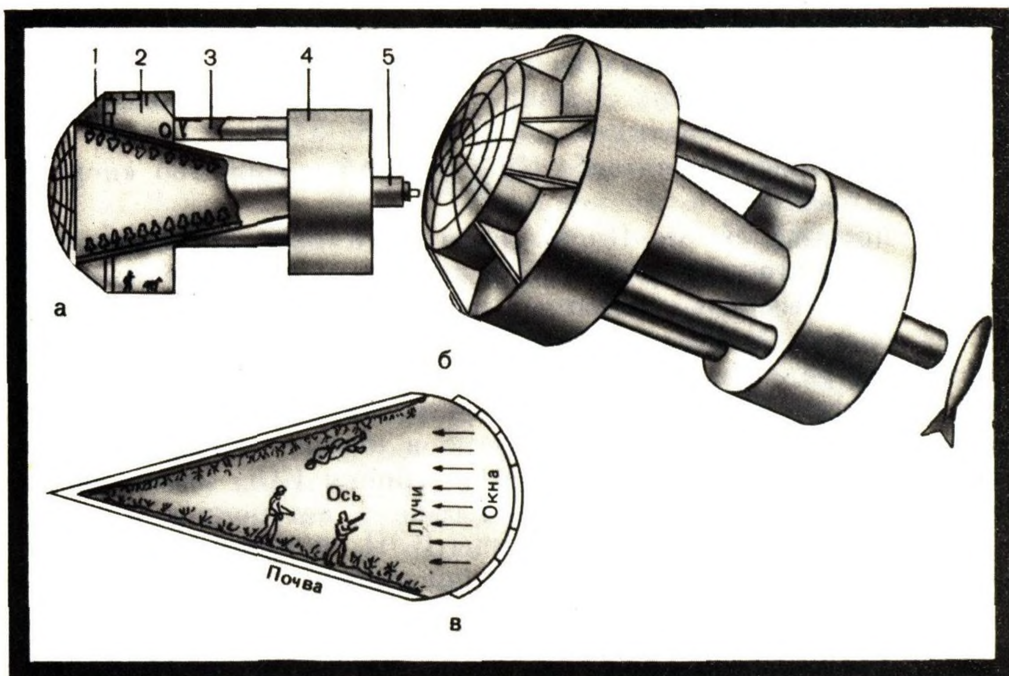
Космическая орбитальная станция по проекту К. Э. Циолковского: а) схема ее устройства: 1 — оранжерея; 2 — жилые помещения и лаборатории; 3 — переходы, 4 — вспомогательные помещения, 5 — причал, б) внешний вид станции; в) оранжерея.
