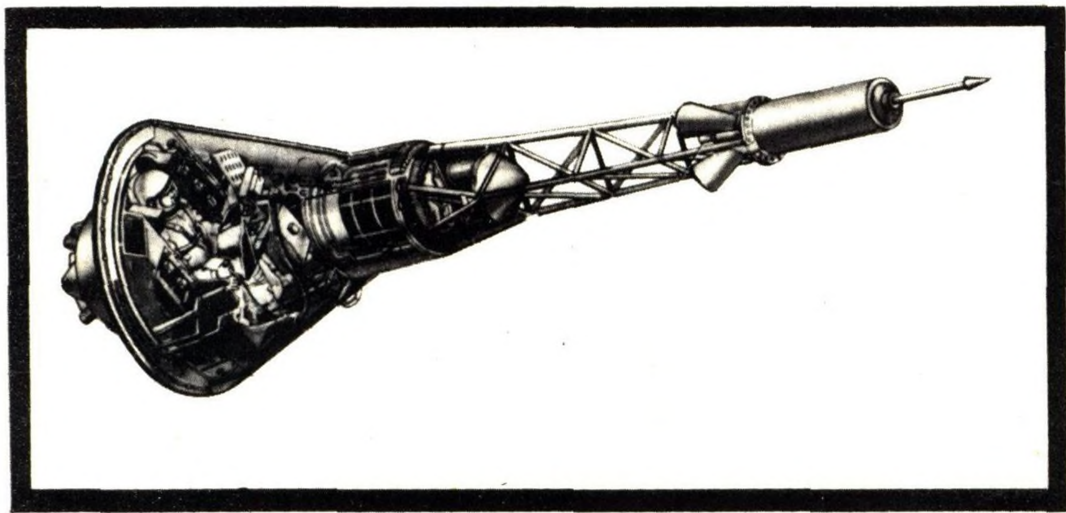
Американский космический корабль «Меркурий».
