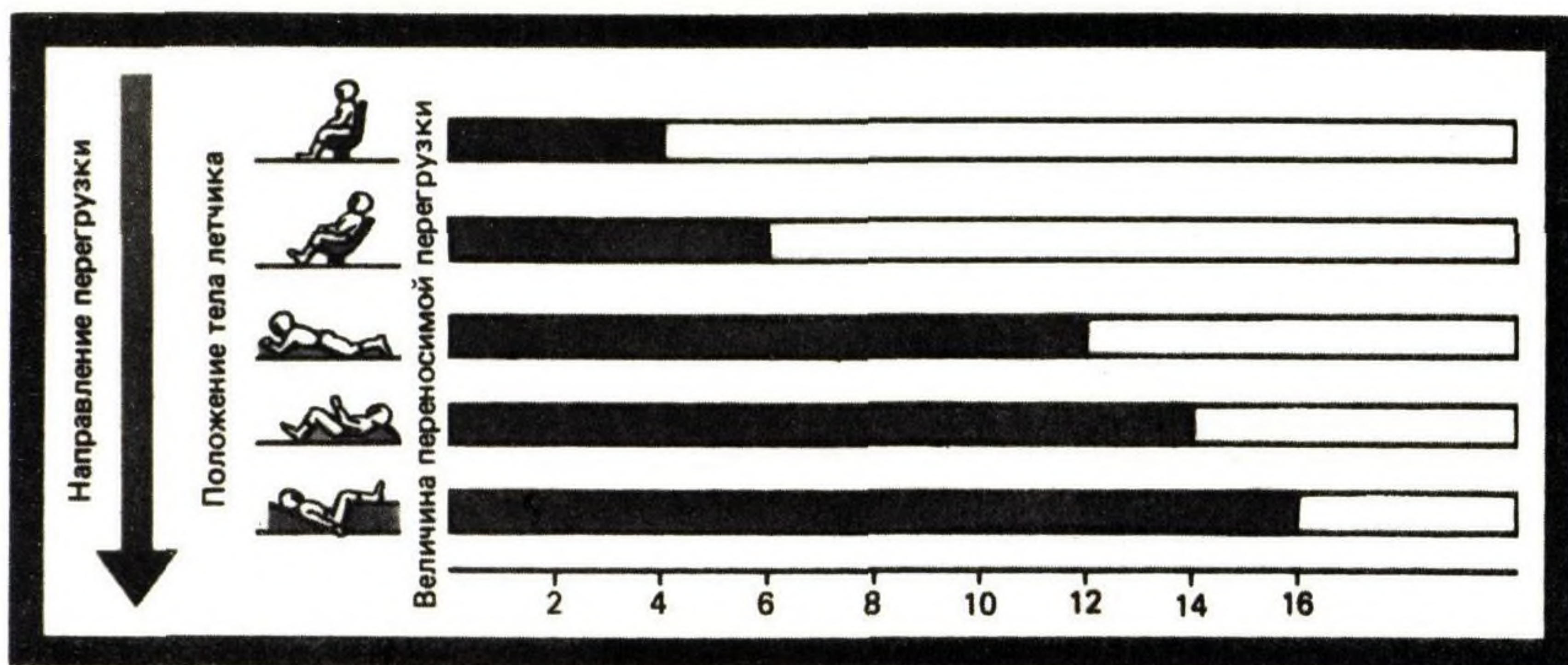
Влияние положение тела на переносимость перегрузки.
