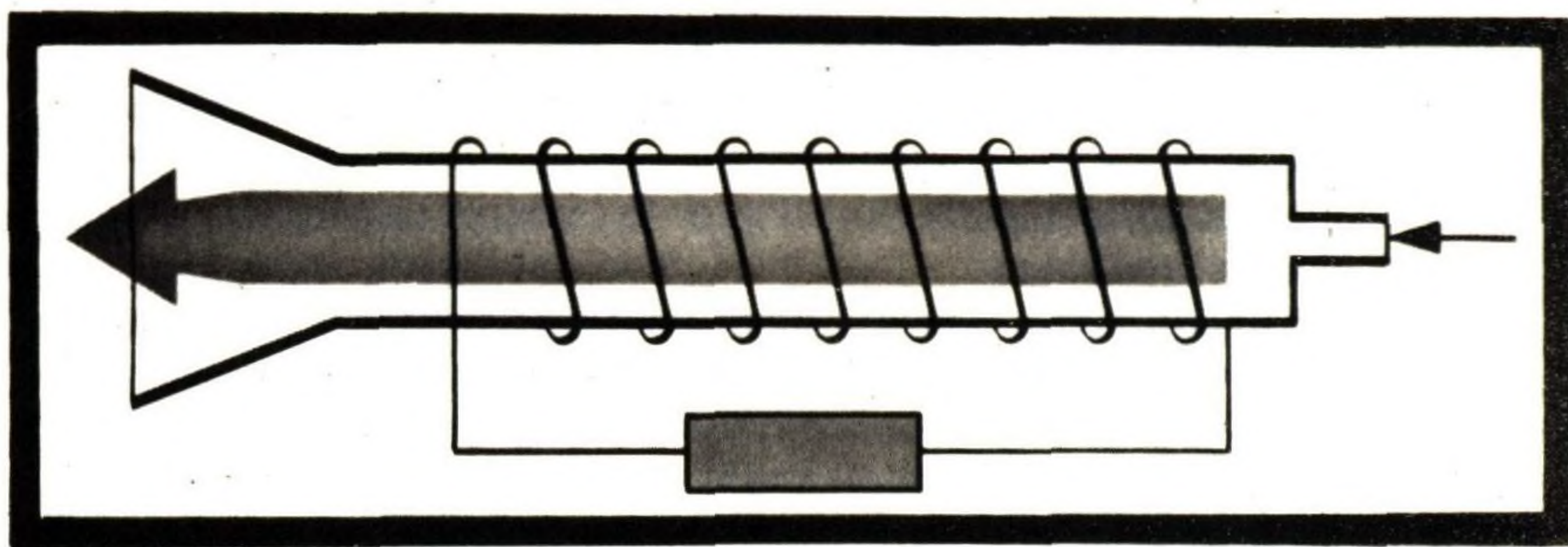
Индукционный плазменный двигатель.
