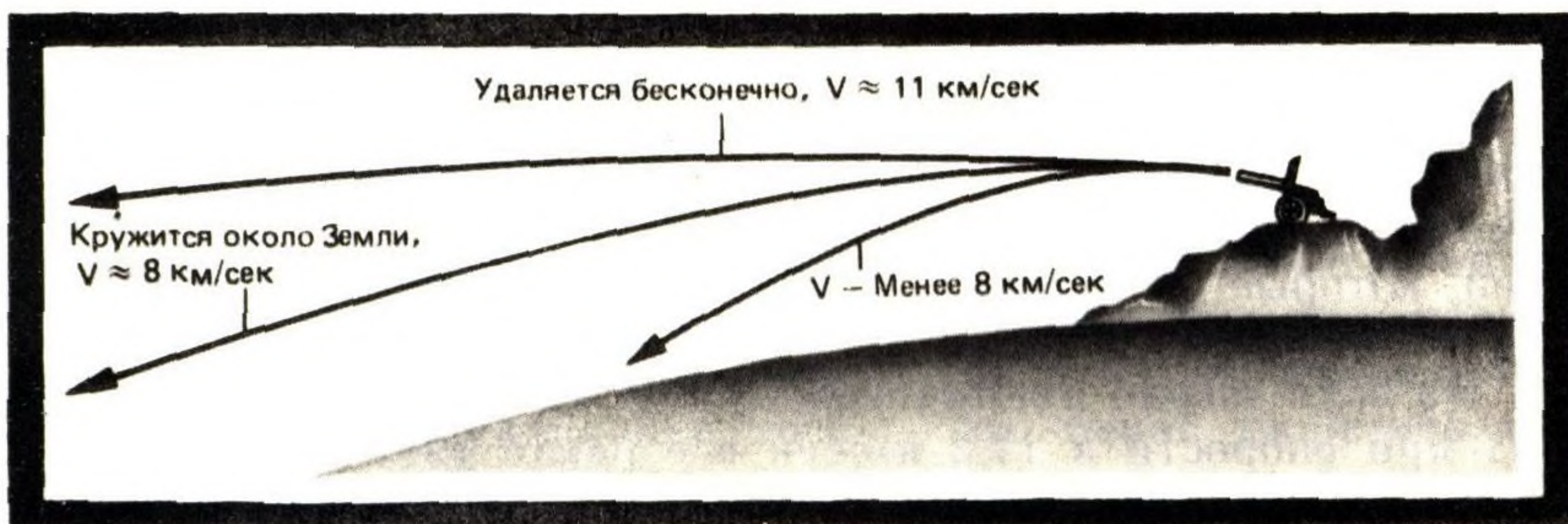
Траектория снаряда «Ньютоновой пушки» при различных начальных скоростях.
