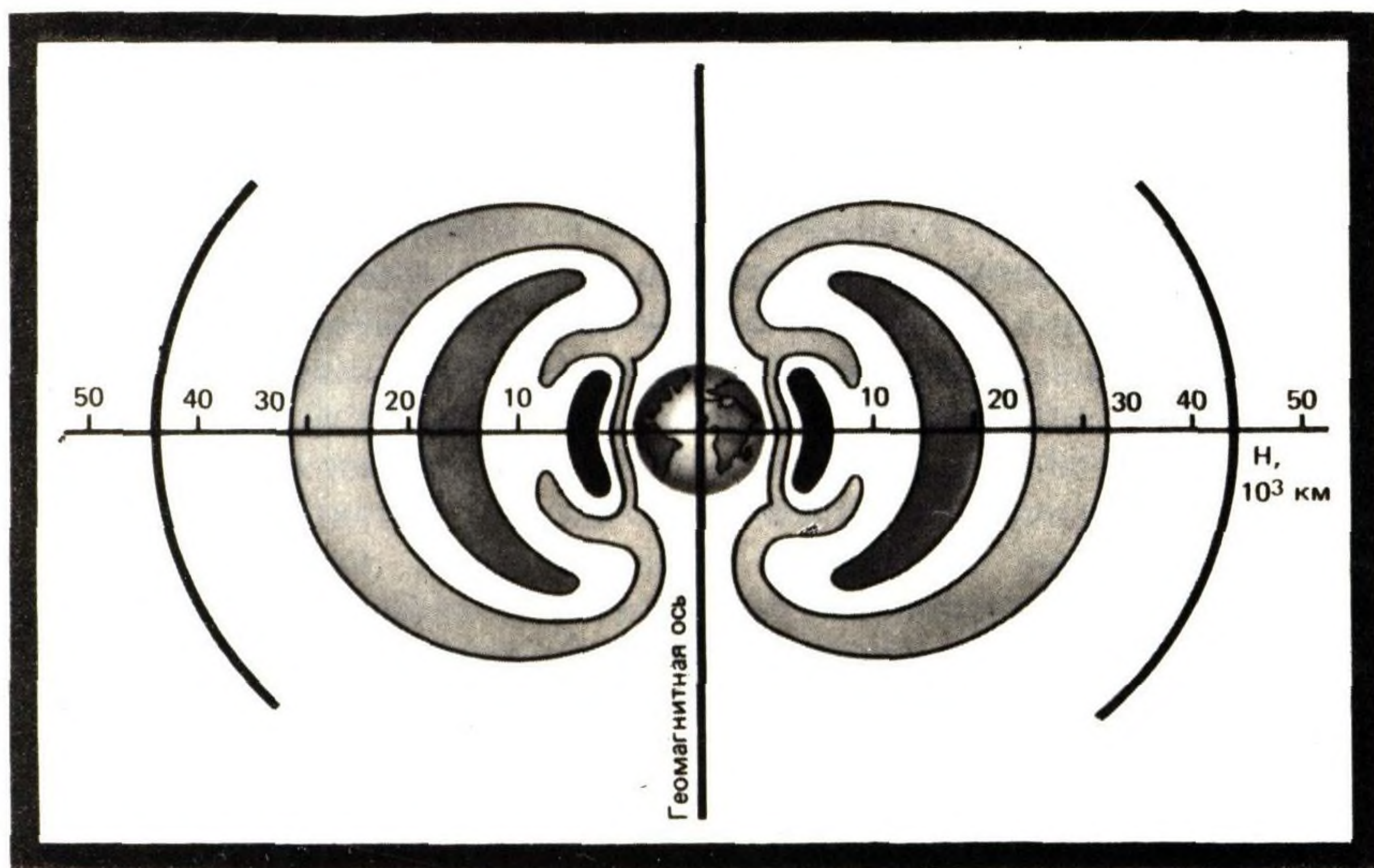
Поперечное сечение поясов радиации.
