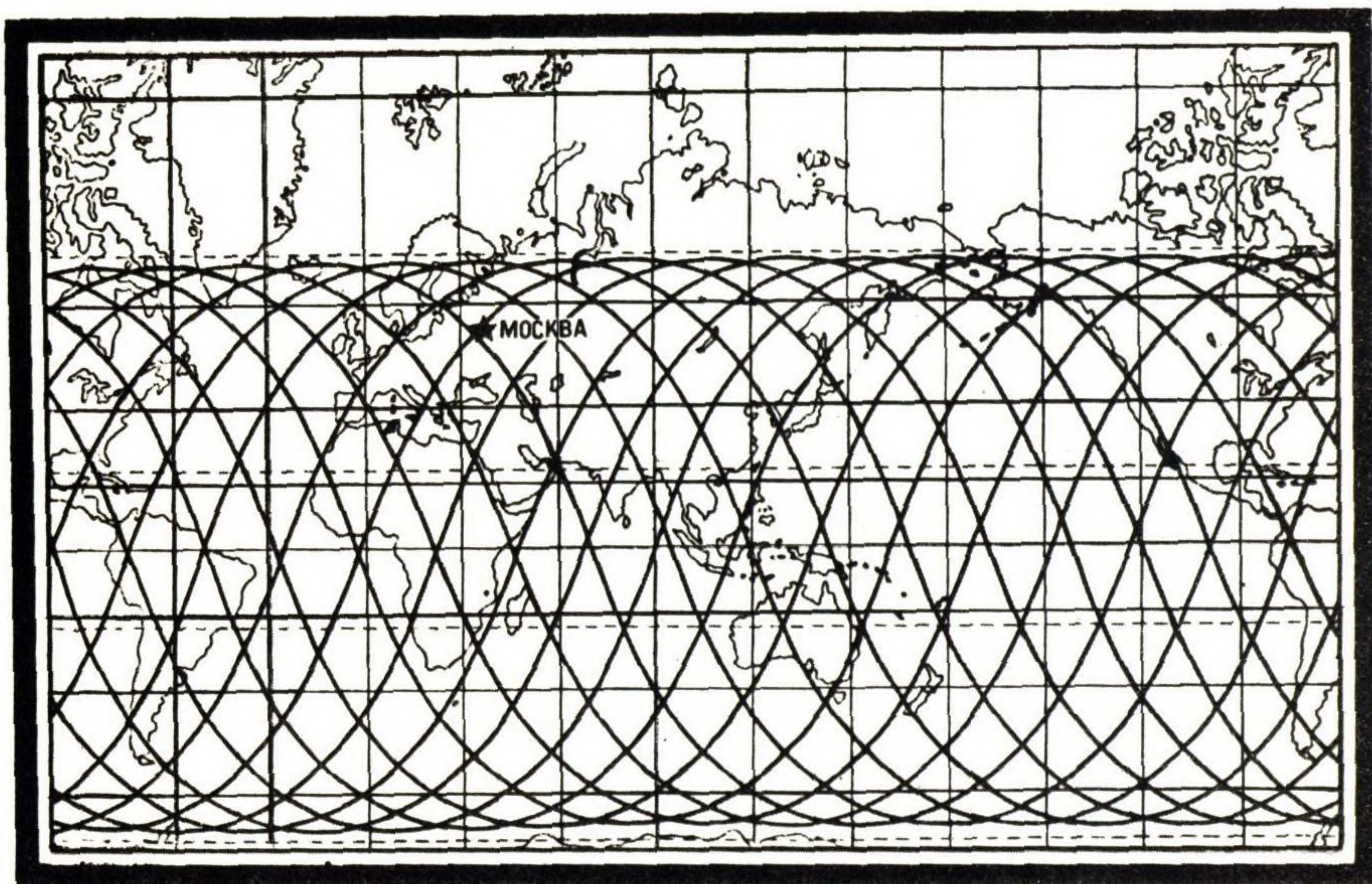
Проекция орбиты спутника на земную поверхность.
