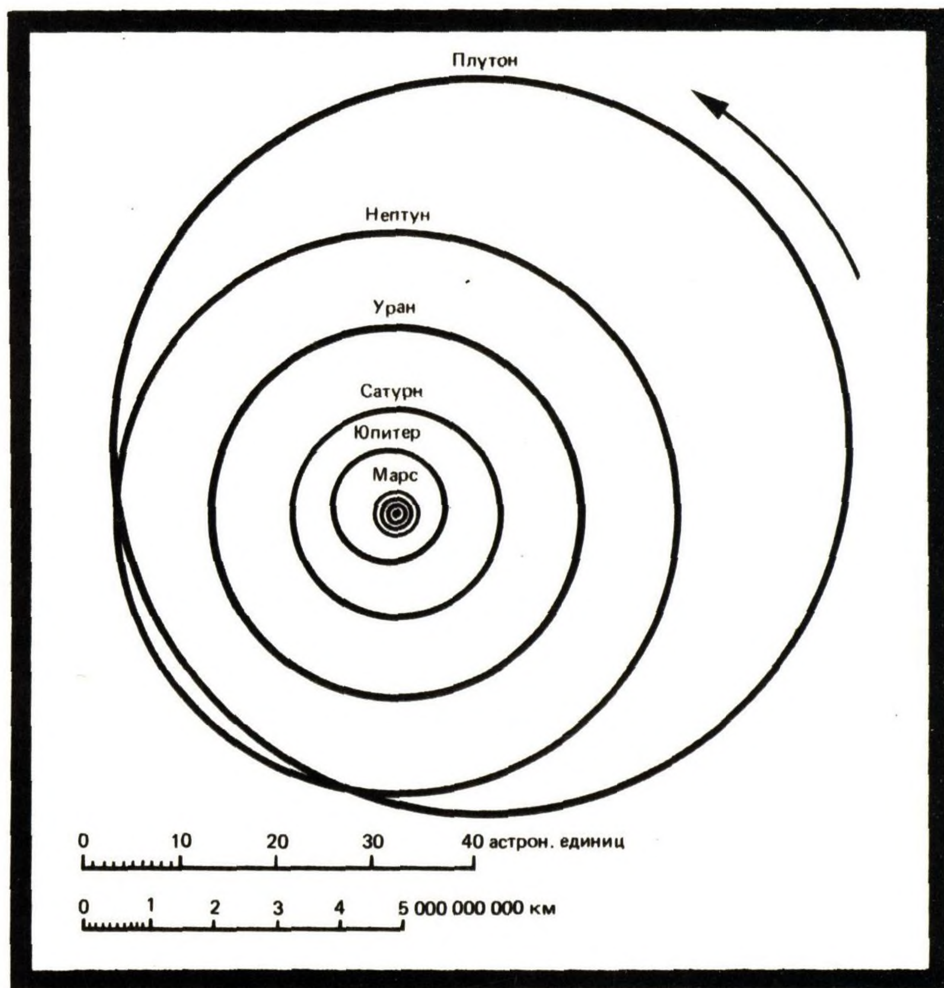
Орбиты главных планет Солнечной системы. Указан масштаб.
